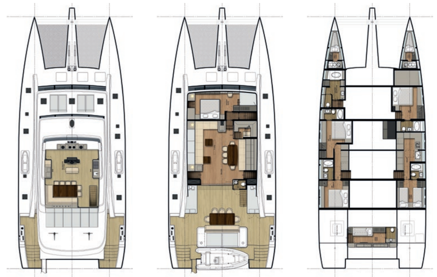
FLYBRIDGE
