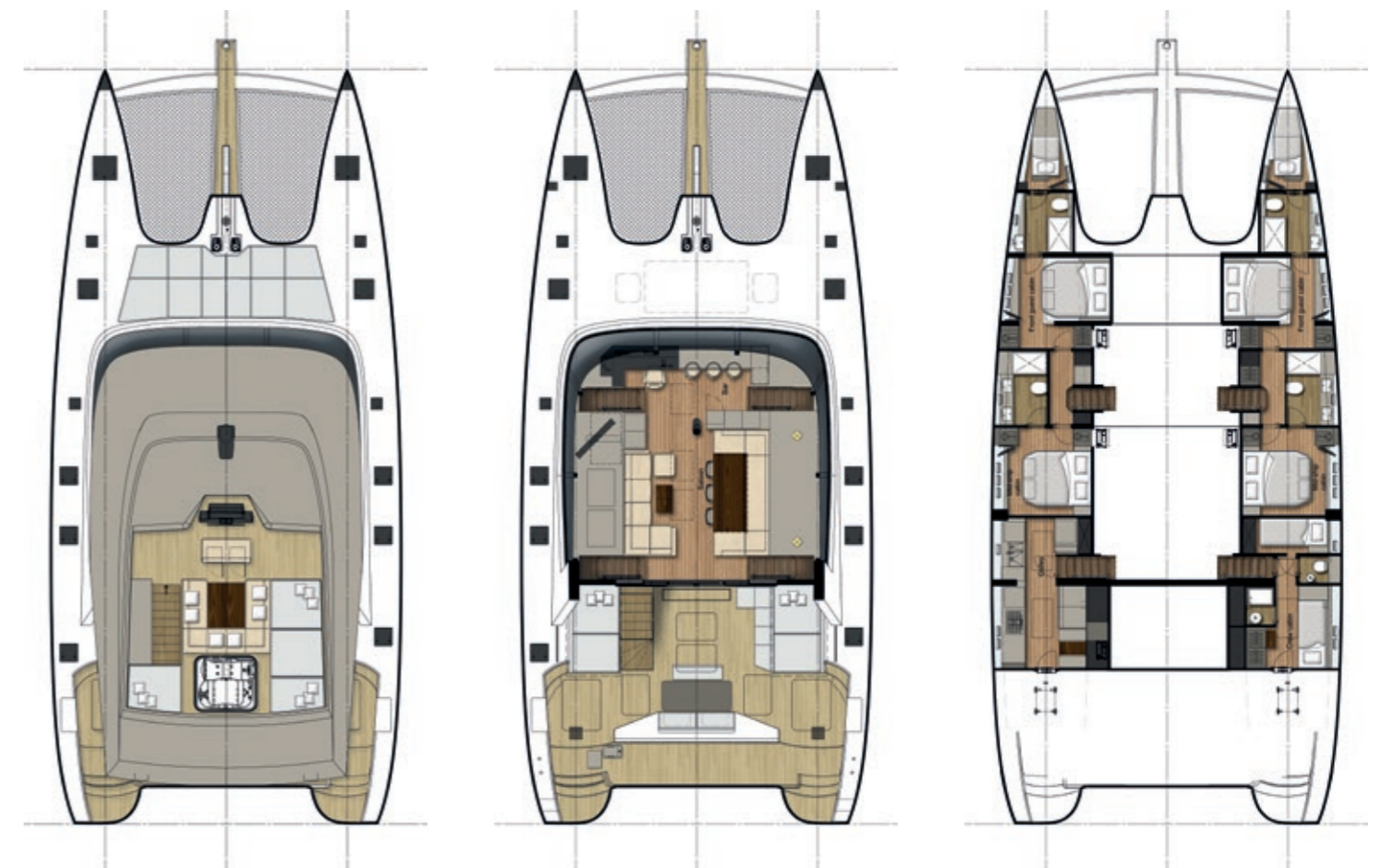
FLYBRIDGE
