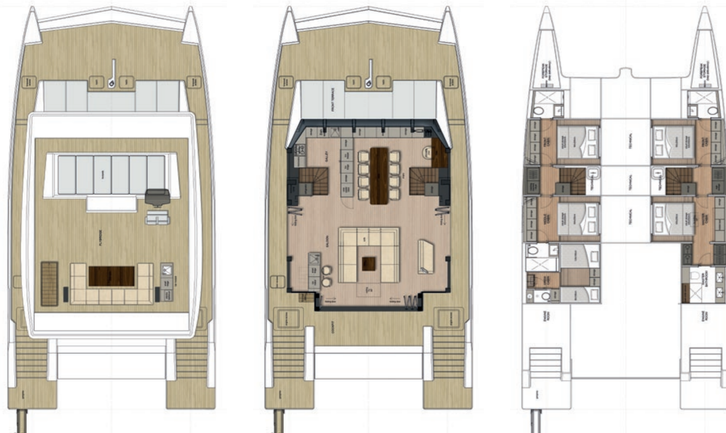
FLYBRIDGE
